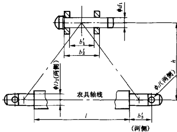
图 6 与农具相关的三点悬挂装置尺寸
