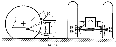
图 4 与拖拉机悬挂点有关的尺寸
