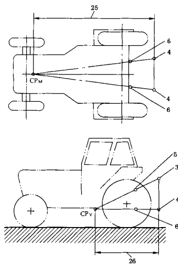
图 7 汇聚距离
