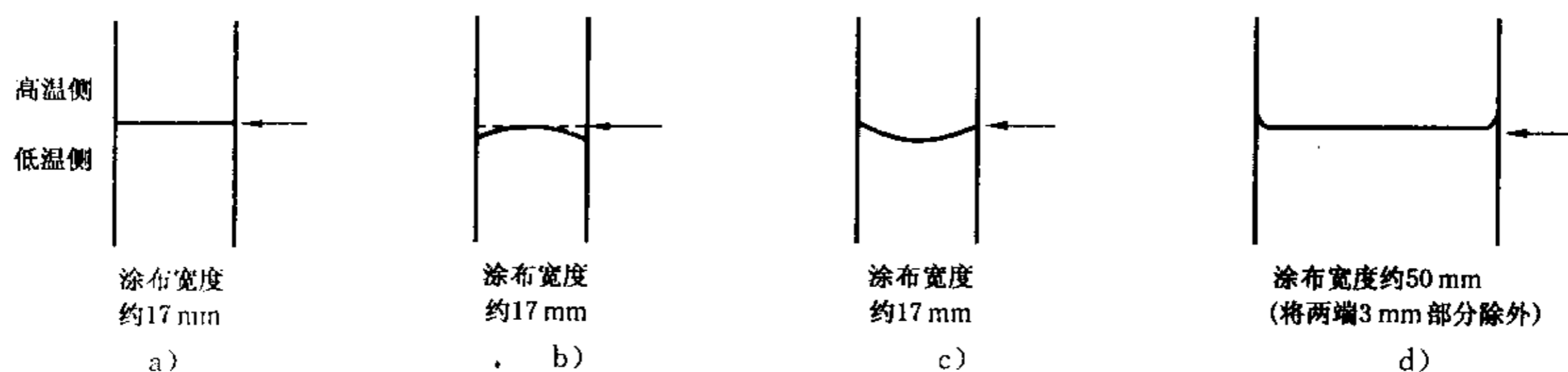
图 4 最低成膜温度的读取方法
